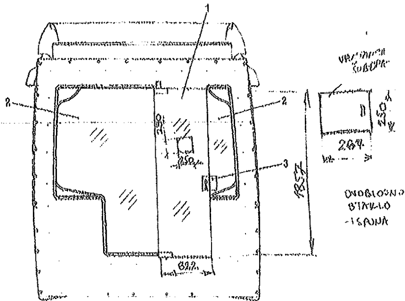
Slika 3-11. Vrata između kabine i salona
